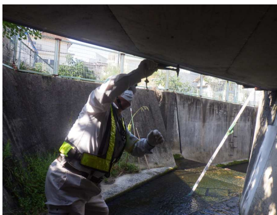
橋梁定期点検状況
