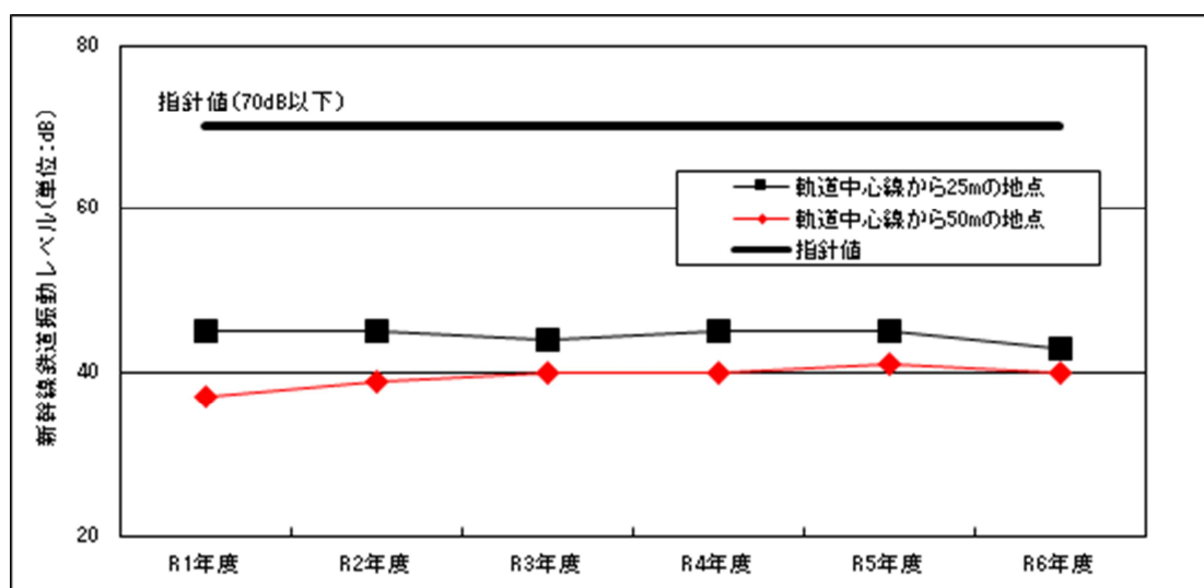
図 4.3 新幹線鉄道振動調査結果の経年変化
