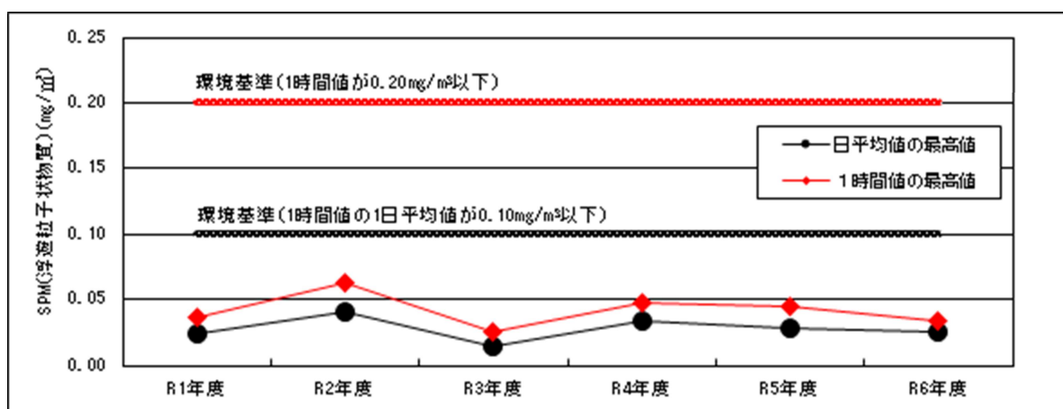
図 1.3 浮遊粒子状物質 (SPM) 濃度の経年変化 (日平均値の最高値及び1時間値の最高値)
