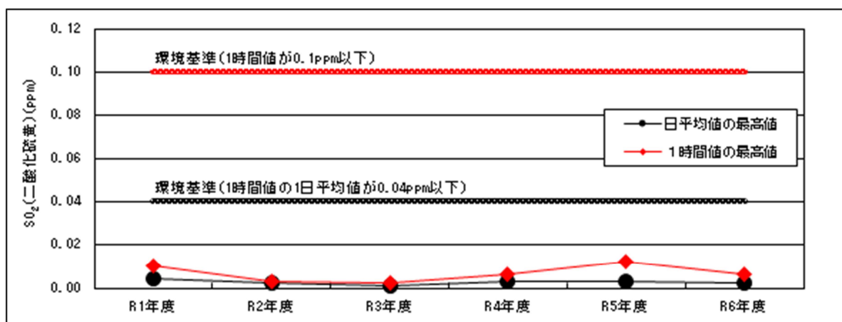
図 1.4 二酸化硫黄 (SO₂) 濃度の経年変化 (日平均値の最高値及び1時間値の最高値)
