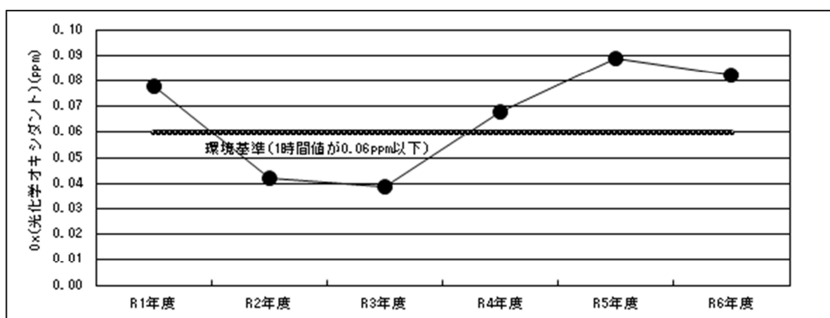
図 1.5 光化学オキシダント (Oₓ) 濃度の経年変化 (1時間値の最高値)
