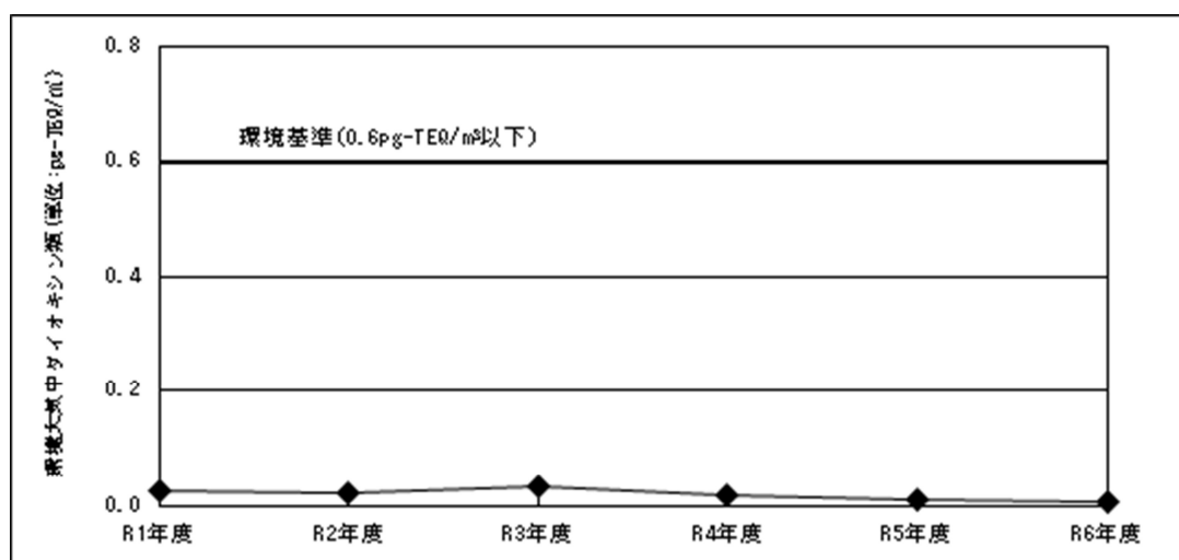
図 5.2 大気中のダイオキシン類調査結果の経年変化
