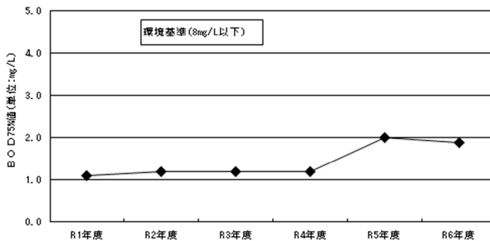
図 2.2 水質（府中大川のBOD（75%値））調査結果の経年変化
