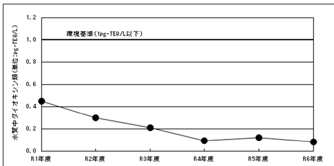
図 5.3 河川水中のダイオキシン類調査結果(夏季)の経年変化
