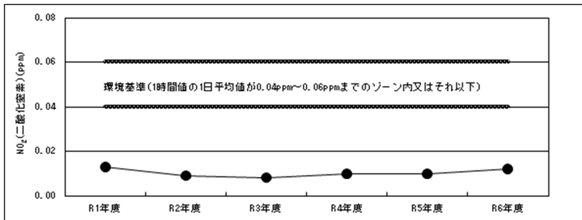
図 1.2 二酸化窒素 (NO 2 ) 濃度の経年変化 (日平均値の最高値)
