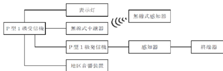
図10の 2 - 1 無線式自動火災報知設備の構成図例
