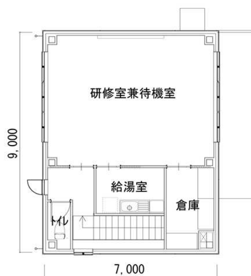
2階平面図
