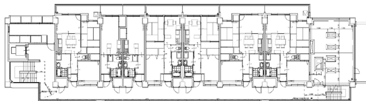
4・5階平面
