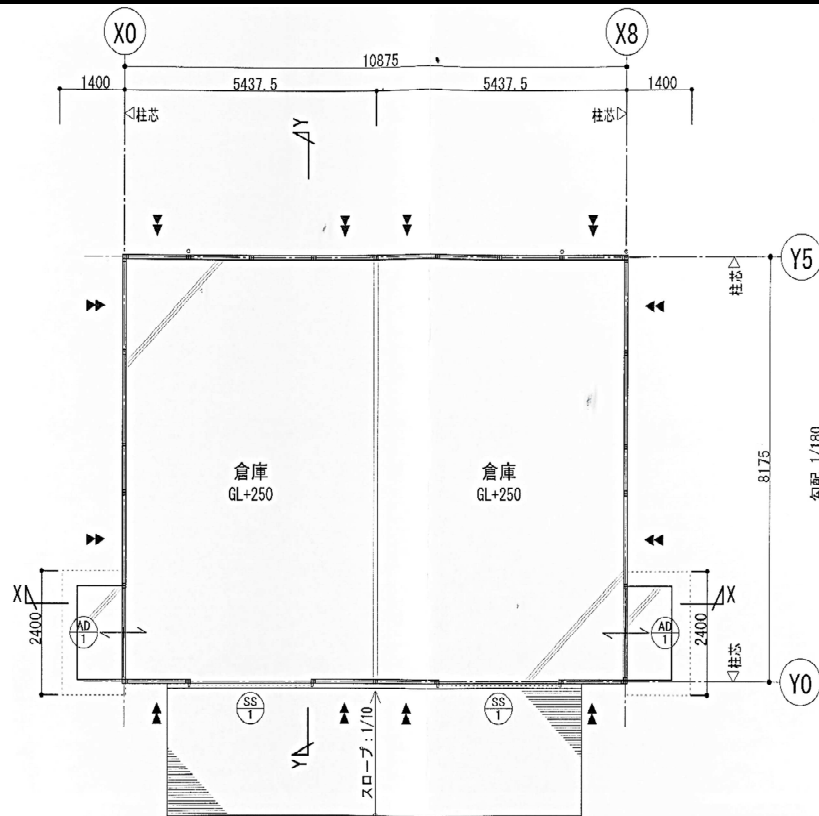
平面図
