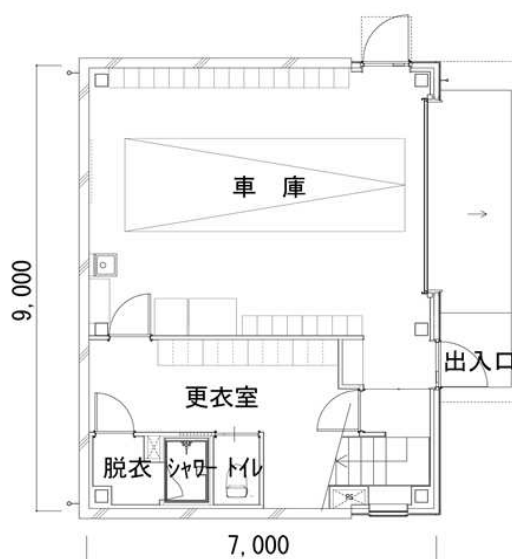
1階平面図
