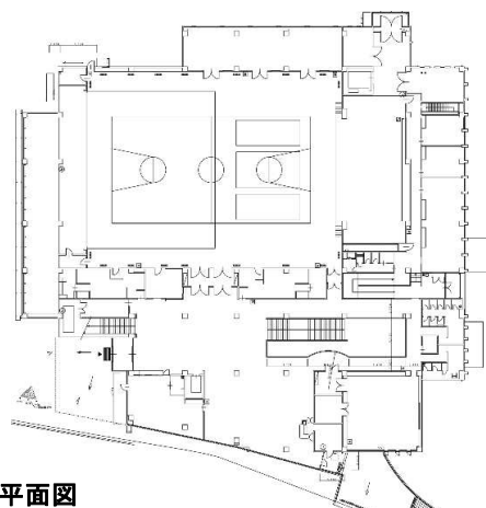
4階平面図
