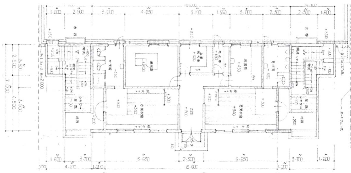
平面図
